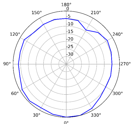
2.4GHz (Vertical)
